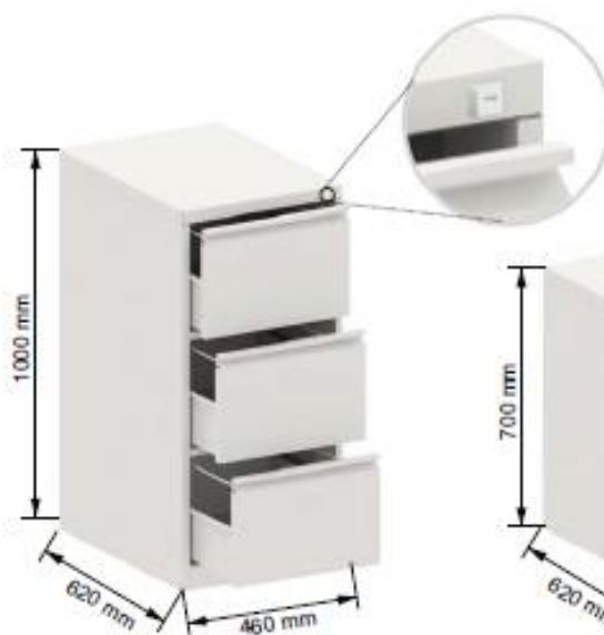
B 3 ÇEKMECELİ 3 DRAWER
