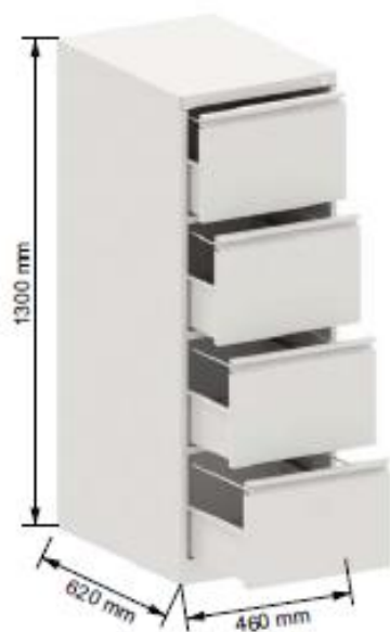
A 4 ÇEKMECELİ 4 DRAWER
